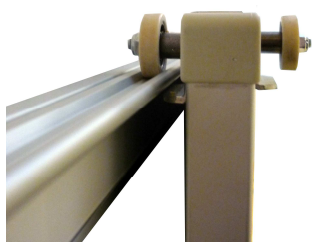
Führung der oberen Schiene
